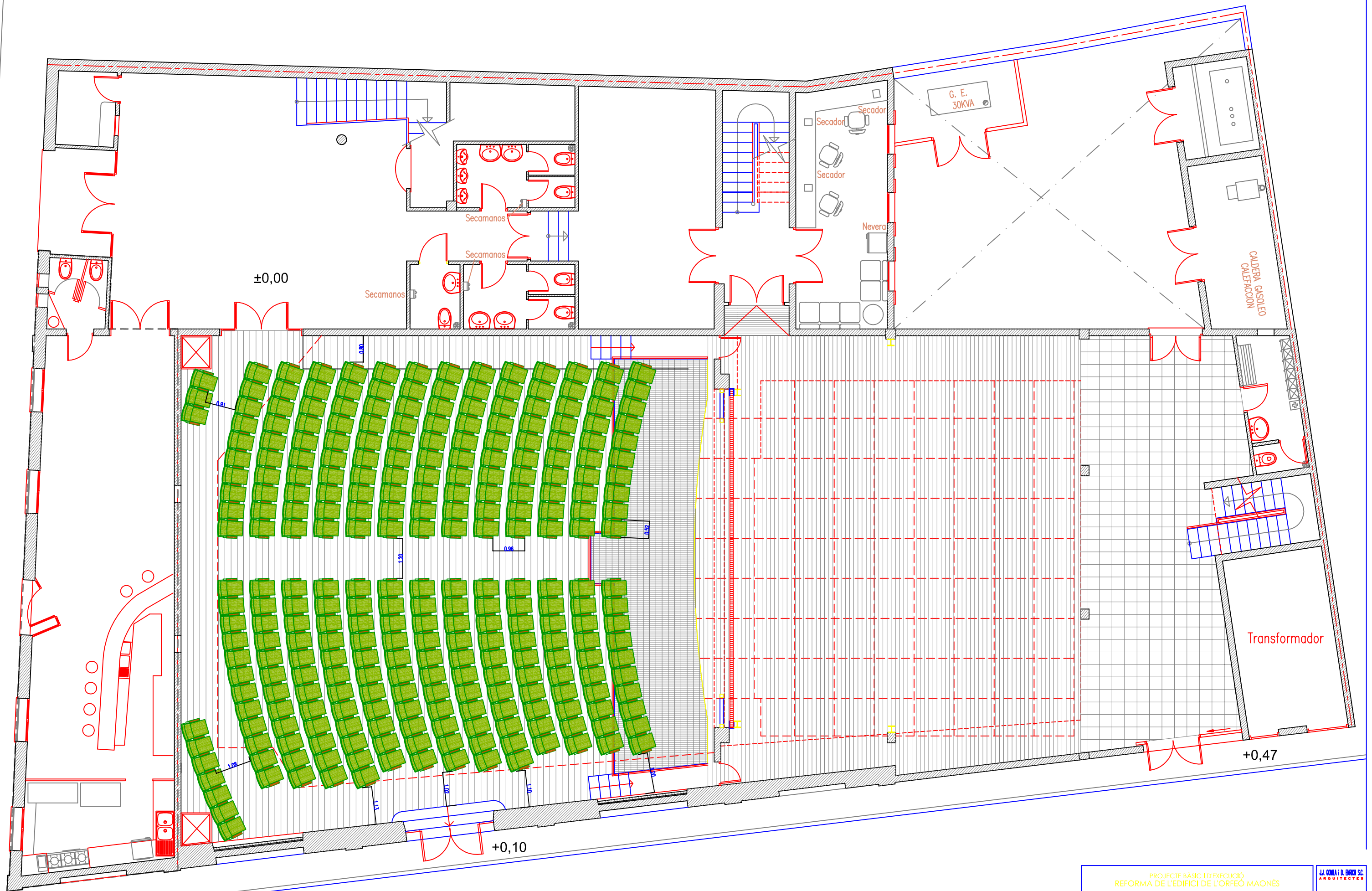
PLANTA BAJA 553.89m2 (Sin Patio)
